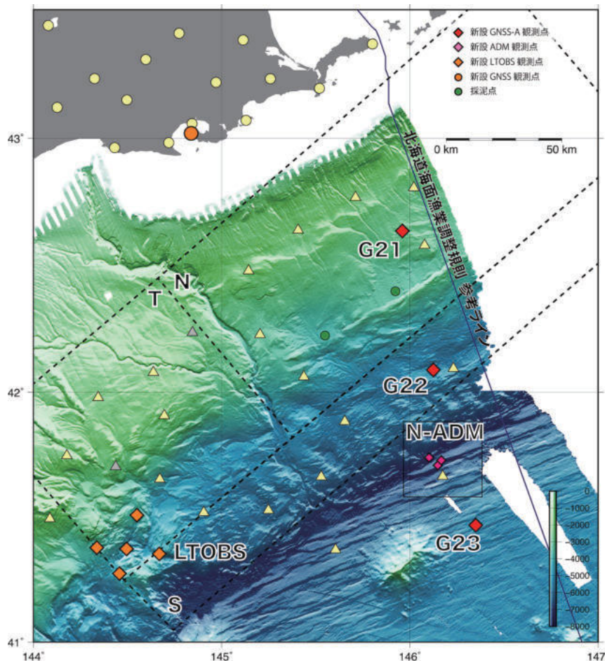
図2. 2019年7月に千島海溝根室沖に設置した海底測地観測点の配置図。赤ひし形がGNSS-A観測点, ピンク色ひし形がADM(海底間音響測距)観測点を示します。オレンジ色ひし形が海底地震計のアレイ観測網(LTOBS)を示します。図中破線の四角は, 17世紀に発生したと考えられている超巨大地震の断層面を示します。黄色三角印は, 防災科学技術研究所が展開する日本海溝海底地震津波観測網(S-net)の観測点を示します。
