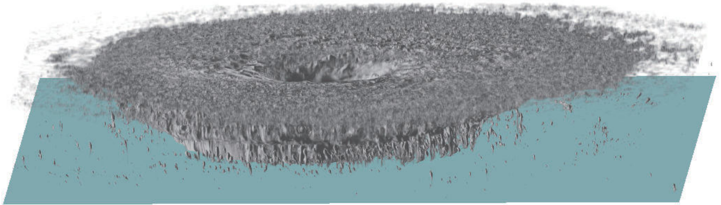
図1. 台風全域の超高解像度シミュレーションにより再現された雲
