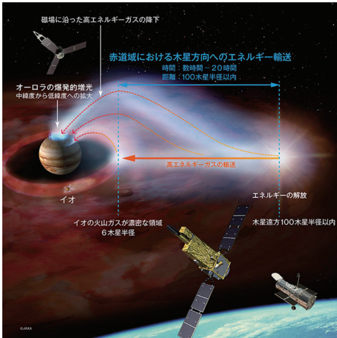
図. 私達が「ひさき」やハッブル宇宙望遠鏡の協調観測で明らかにした木星磁気圏のエネルギー輸送過程 (©JAXA)
