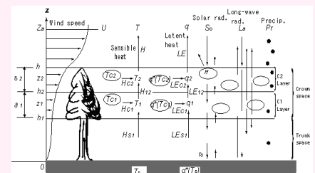
【図7】陸面過程モデル 2LM の概念図
