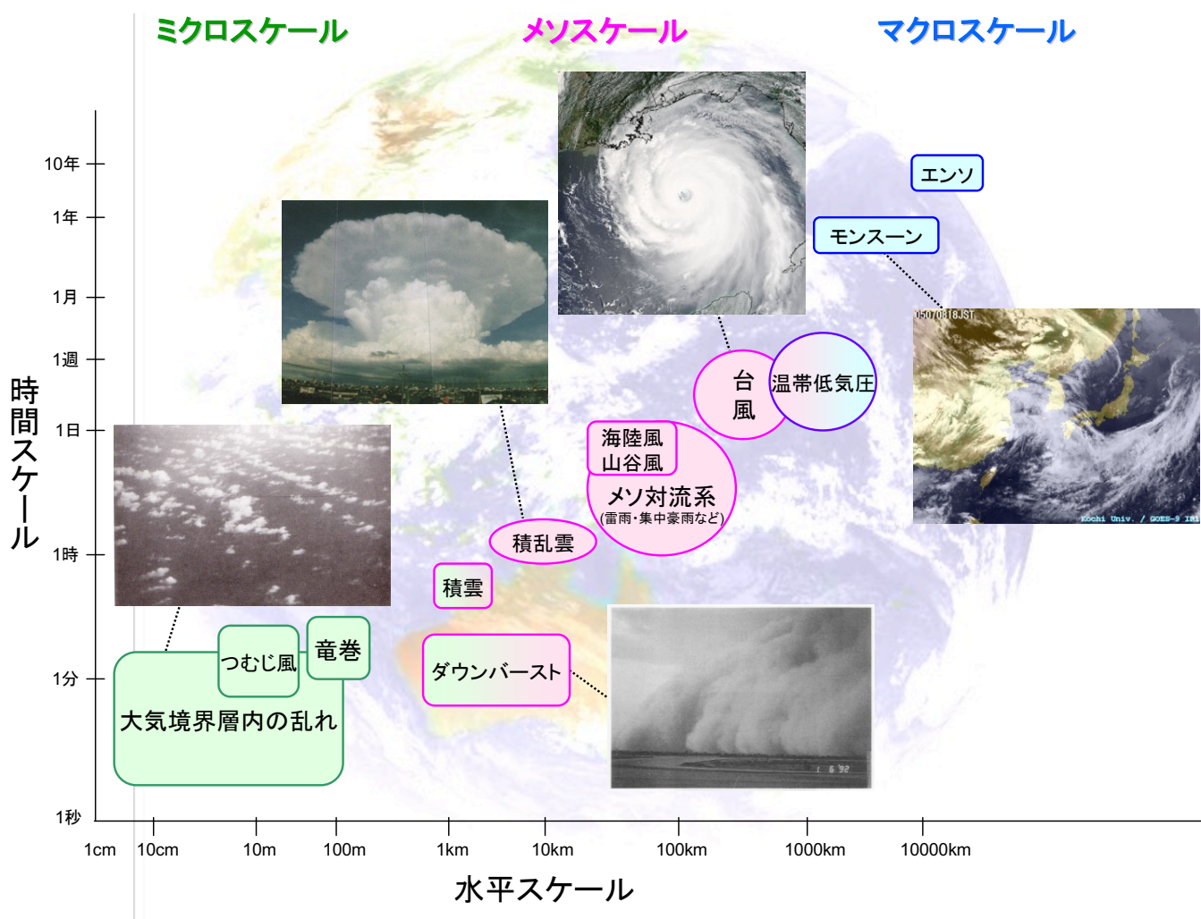
【図1】大気の運動の時間・空間スケール（『一般気象学』の中の図を変更）
