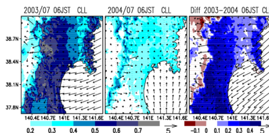
【図 6】 (左) 東北沖のヤマセ、(右) 2003、2004 年 7 月の再現実験で得られた下層雲量。朝 6 時における 1 ヶ月平均値を示す。それぞれ左から 2003 年の再現結果、2004 年の再現結果、2003 年と 2004 年の差。雲量は 0-1 の値。0 で雲無し、1 で全面雲で覆われていることを表す。
