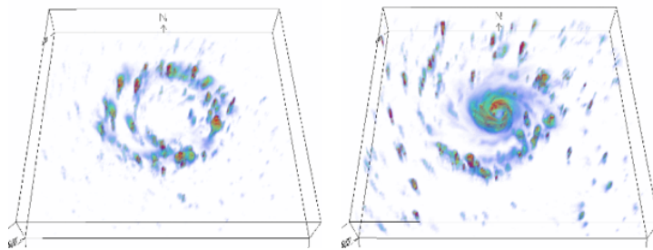
【図 5】 数値実験で再現された台風の雲の3次元分布。暖色系ほど雲の濃い部分を示す。表示領域は400km四方。(図左)は計算開始から12時間後、(図右)は60時間後を示す。
