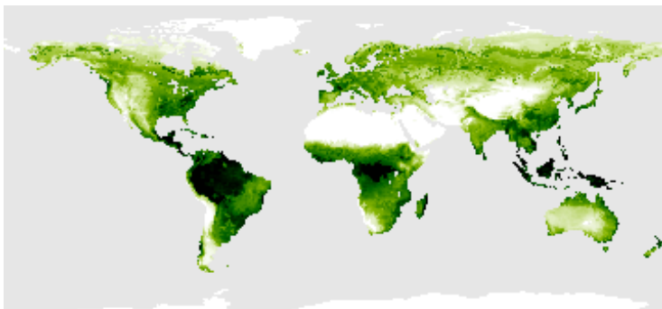
【図8】陸域生物圏モデル BEAMS によって推定された植生の炭素吸収量（1982-2000 年平均値）。アマゾンや東南アジアなどの赤道付近で高く、高緯度や乾燥地域で低いことがわかつす。
