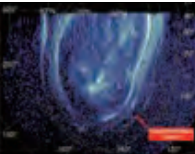
ハッブル宇宙望遠鏡で観測した木星オーロラの極域展開図。衛星エウロパと磁力線でつながる場所にスポット状のオーロラ発光が確認できる。
