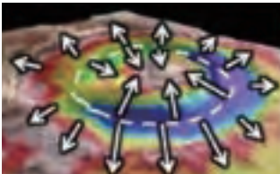
(左)火星周回探査機による近赤外分光データの解析から明らかにした風の流れ。(右)2024年に打ち上げ予定の火星探査機MMX
