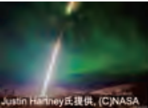
(左)脈動オーロラとともに降ってきていると考えられているキラー電子の想像図。(右)LAMPロケット発射の瞬間 (©脈動オーロラプロジェクト)
